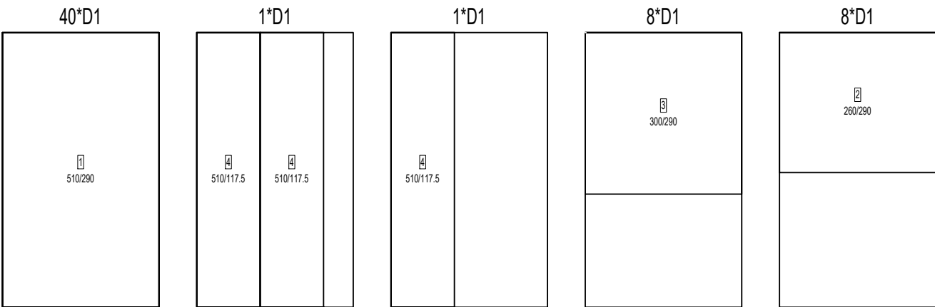
Schita taiere plase
