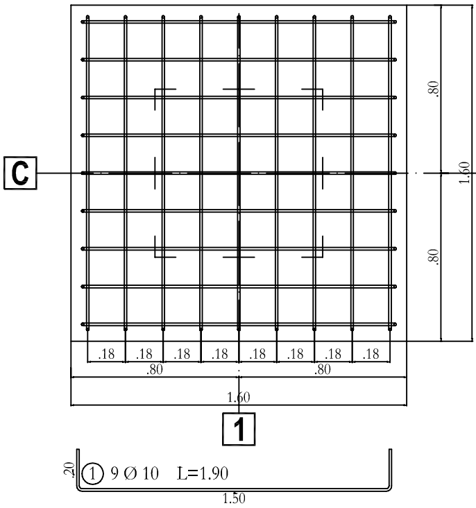
Secțiunea 1-1
